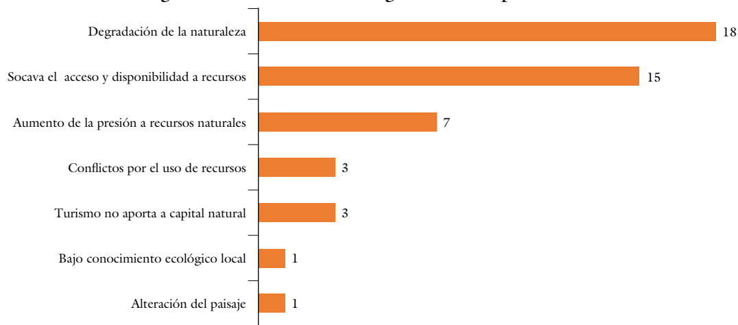
Figura 6. Transformaciones negativas en el capital natural
