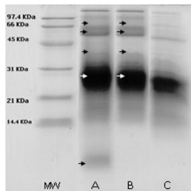
Figura 4. SDS-PAGE revelados con azul de Comassie del veneno de B. asper después de 30 minutos de incubación con los extractos en una relación de 1:10. MW: Marcadores de peso molecular 97.4, 66, 45, 31, 21 y 14.4 KDa. A: H. psittacorum . B: H. rostrata . C: Veneno completo. Las flechas señalan las bandas de proteína, donde se observan cambios en relación con el veneno solo.
